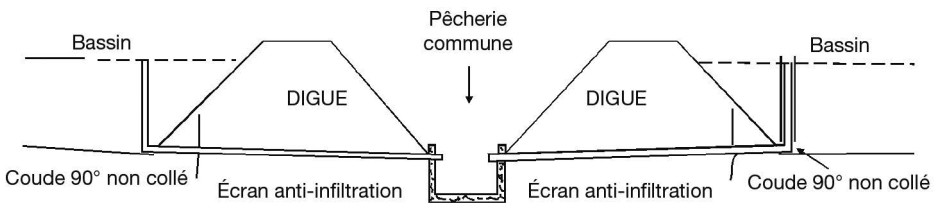
Figure 4. Bassins avec bondes basculantes en PVC et pêcherie commune.
