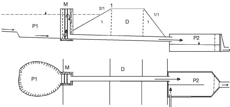
D : digue – M : moine du type Herrguth P1 : poêle de l'étang – P2 : pêcherie avec arrivée d'eau fraîche
