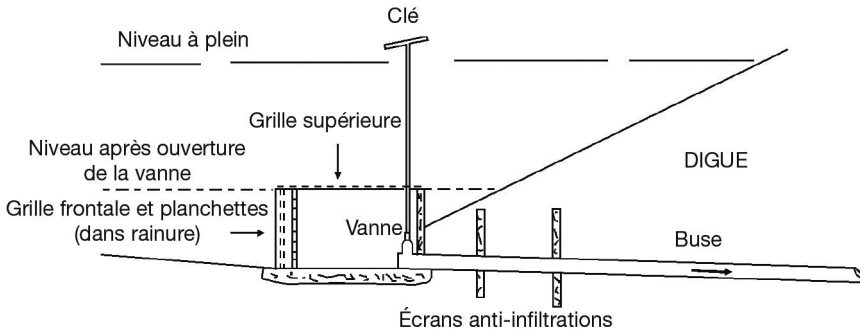
Figure 3. Moine à vanne. Schéma de l'installation.
